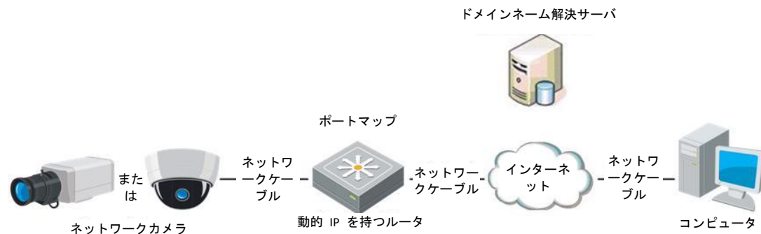
図 2-12 通常のドメイン名の解決
