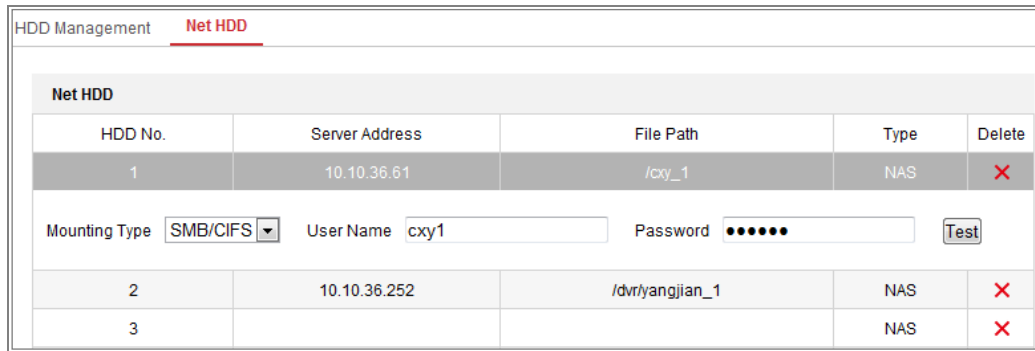
図 10-6 ネットワークディスクの追加
