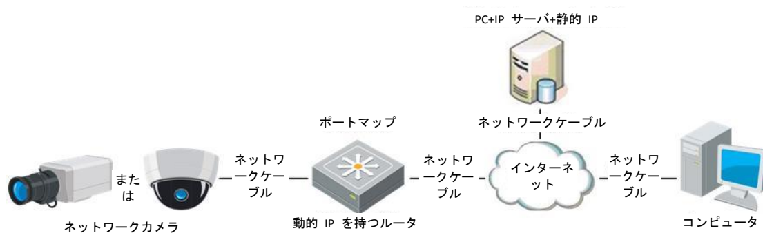
図 2-13 プライベートドメイン名の解決
