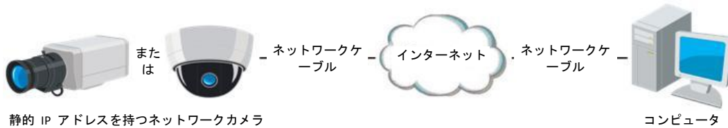
図 2-10 静的 IP を持つカメラによる直接アクセス
