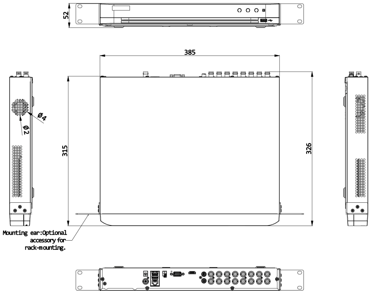
scale/1:1;Unit/mm
