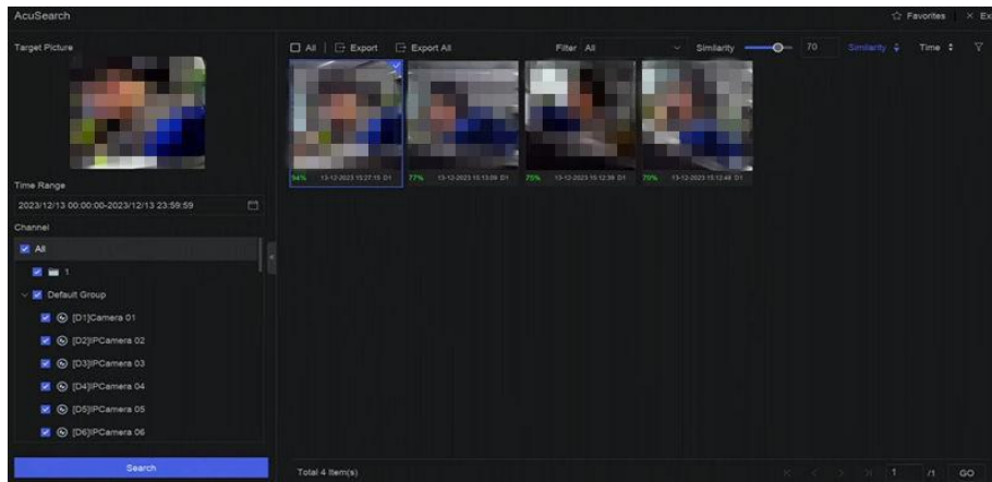
図15-2 AcuSearchの結果
