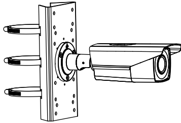
DS-1275ZJ-SUS ポール取付金具
