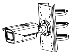
DS-1275ZJ-SUS 垂直ボール取付け金具
