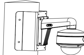
DS-1276ZJ-SUS コーナー金具
